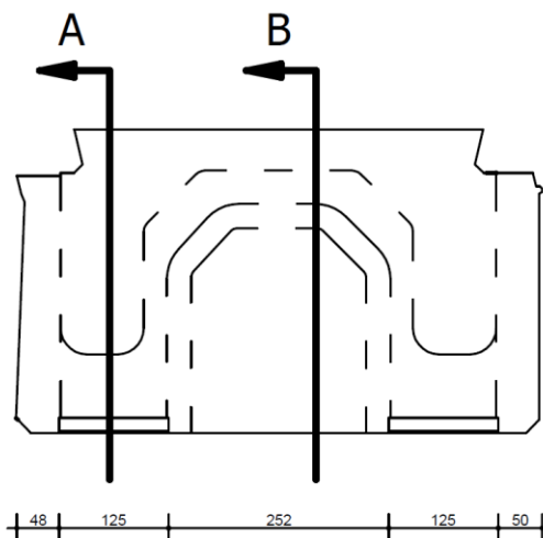
aanzicht kop-paselement
