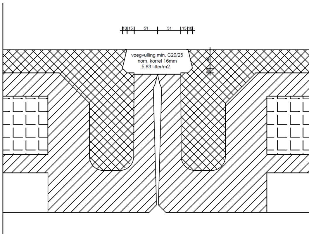
voegdetail
