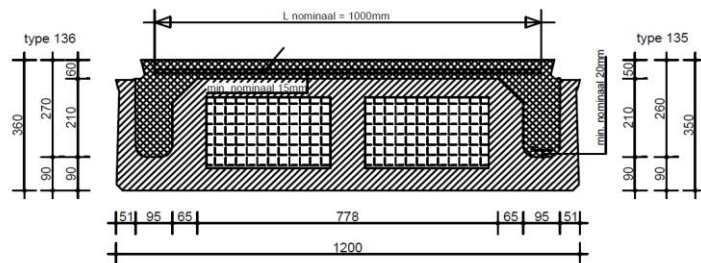
doorsnede vloerelement type 135/136 Rc=5,0 m2K/W
