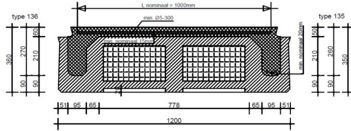
doorsnede vloerelement type 135/136 Rc=4,5 m2K/W
