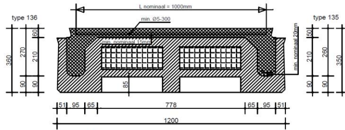
doorsnede vloerelement type 135/136 Rc=3,7 m2K/W
